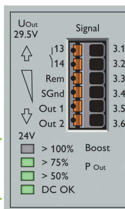
QUINT4の前面
