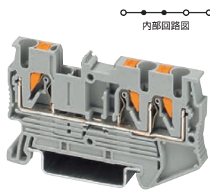
3線式 (1対2) ※ 弊社呼称：TWIN
