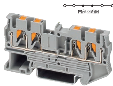
4線式 (2対2) ※ 弊社呼称：QUATTRO
