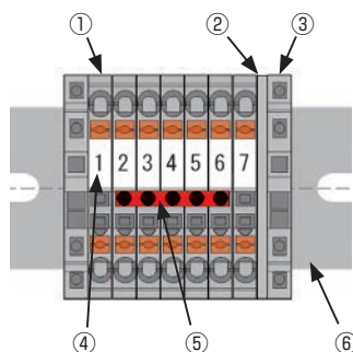
基本的な部品構成 ※上図は当社専用組立端子台ソフト「CLIPPROJECT」で作成
